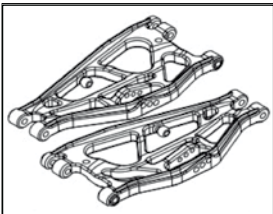
6121 Querlenker hinten rear suspension arms 2set
