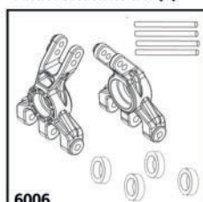
6006 Radträger hinten (2)
